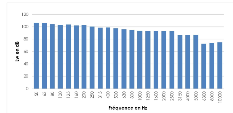
Graphique 4. Spectre de puissance acoustique par bande de tiers d'octave : vitesse de 7 m/s (à la hauteur standardisée de 10 m) SIEMENS GAMESA SG 6,0-155 – 6 MW
