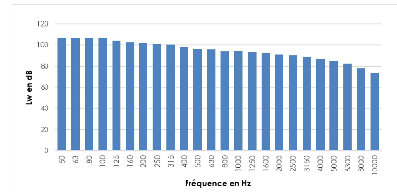
Graphique 3. Spectre de puissance acoustique par bande de tiers d'octave : vitesse de 7 m/s (à la hauteur standardisée de 10 m) NORDEX N149 4,8MW
