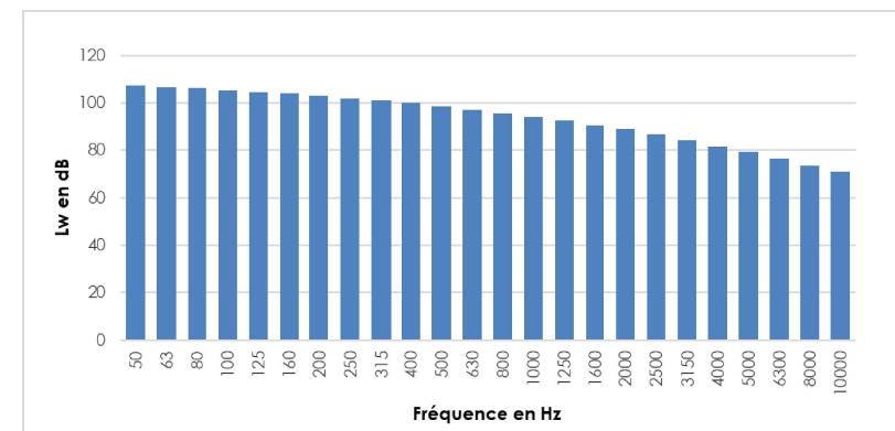
Graphique 1. Spectre de puissance acoustique par bande de tiers d'octave : vitesse de 7 m/s (à la hauteur standardisée de 10 m) VESTAS V150 – 4.2 MW
